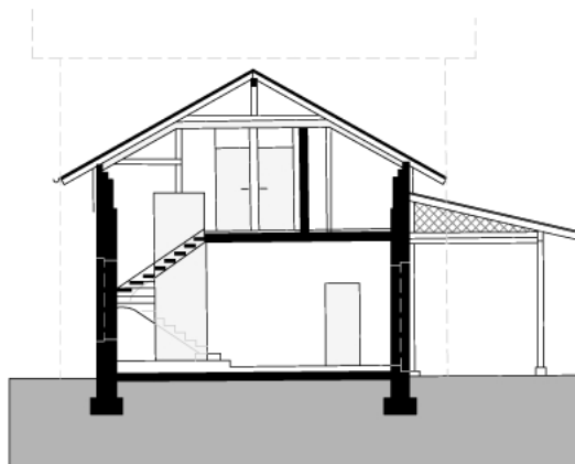
SCHNITT A-A
